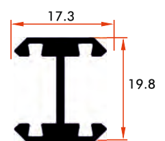
SLP-OPD
