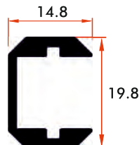
SLP-OPV
