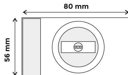
SLP-SLB-4516
