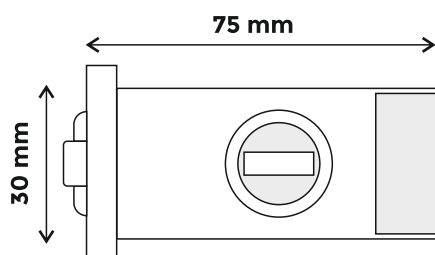
SLP-SLS-4507
